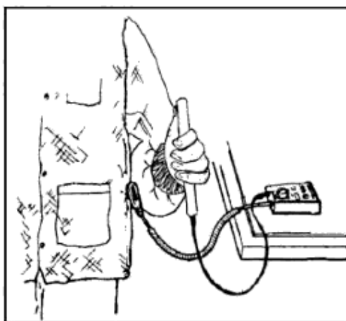
Рисунок 11 — Испытательная сборка — сопротивление системы заземляемой одежды (использование измерителя и ручного электрода при испытании надетой заземляемой одежды)
