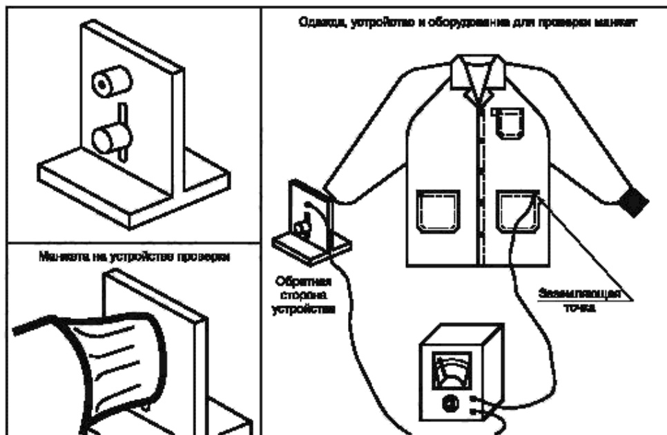
Рисунок 10 — Испытания манжет заземляемой одежды
