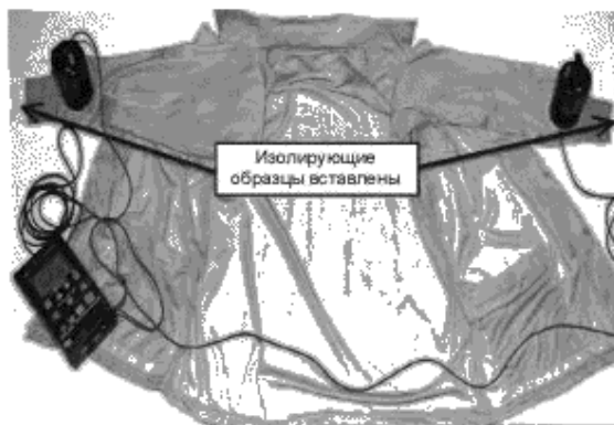
Рисунок 1 — Испытательная сборка — сопротивление «от точки до точки» (процедура «рукав-рукав» с использованием изолирующих вкладок)
