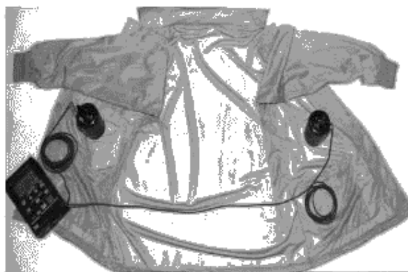
Рисунок 3 — Испытательная сборка — сопротивление «от точки до точки» (процедура «панель-панель» с использованием изолирующей поверхности)
