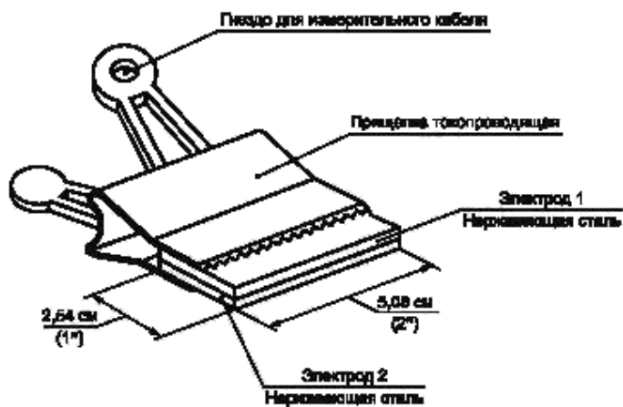
Рисунок 7 — Зажимы/электроды для испытания висящей одежды
