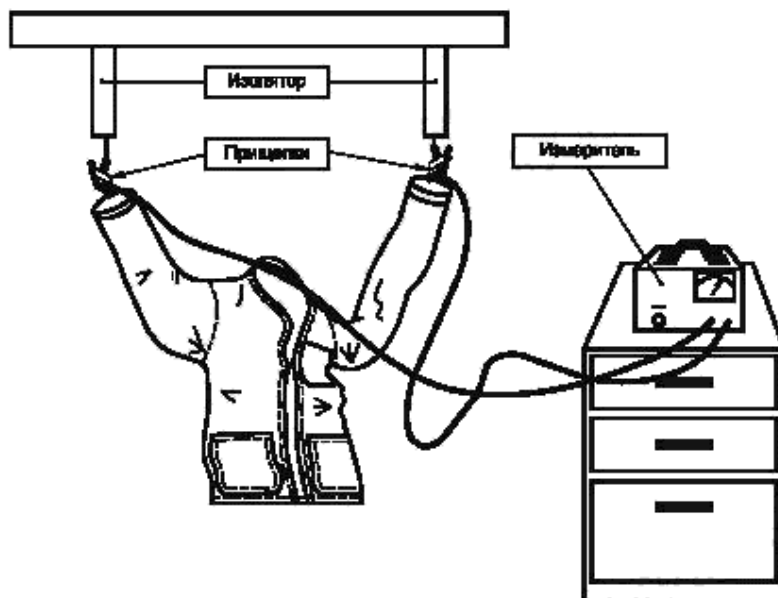
Рисунок 6 — Испытательная сборка — сопротивление «от точки до точки» (процедура «рукав-рукав» с использованием зажимов для подвешивания)
