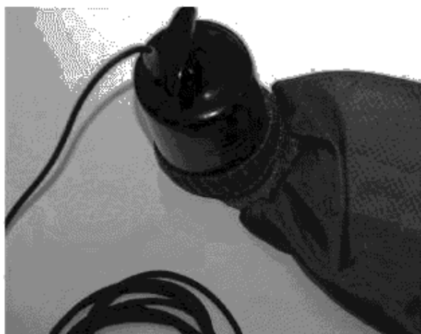
Рисунок 5 — Испытательная сборка — сопротивление «от точки до точки» (детализация вставленного в манжету электрода)
