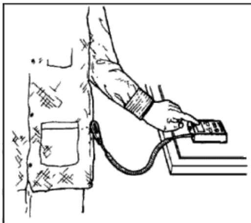
Рисунок 12 — Испытательная сборка — сопротивление системы заземляемой одежды (использование встроенного измерителя при испытании надетой заземляемой одежды)
