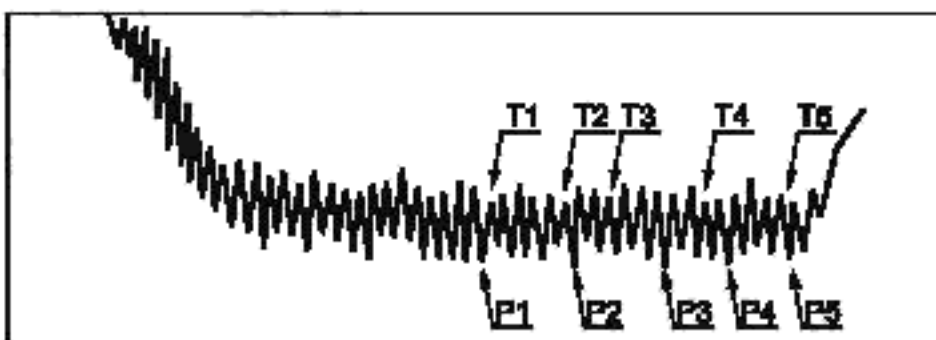
2б — Осциллограмма напряжения человеческого тела отрицательной полярности
