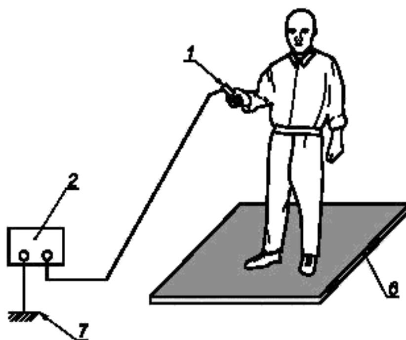
1б — Схема для испытаний установленных полов
