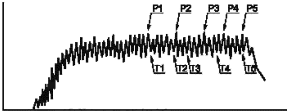
2а — Осциллограмма напряжения человеческого тела положительной полярности
