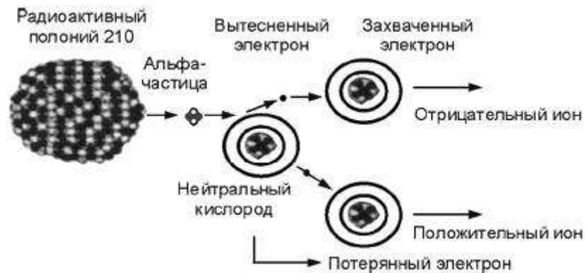
Рисунок 9 - Ионизация альфа-излучением
