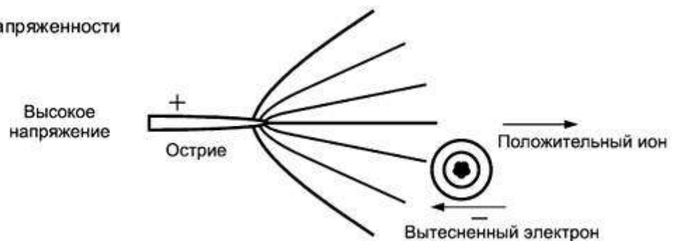
Рисунок 10 - Коронная ионизация - положительная
