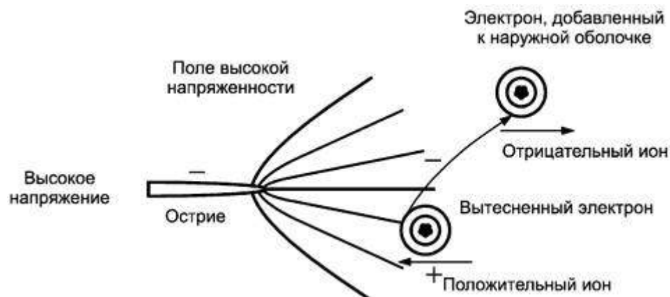
Рисунок 11 - Коронная ионизация - отрицательная
